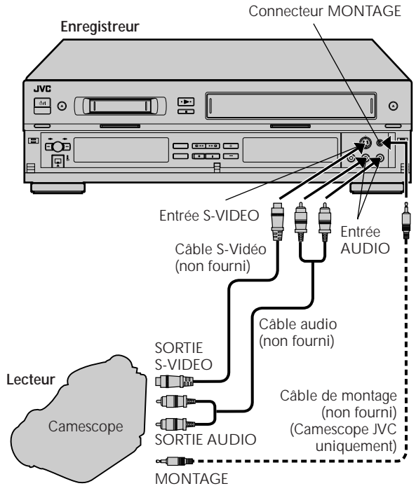
B Si le caméscope a un connecteur de sortie S-VIDEO ...
