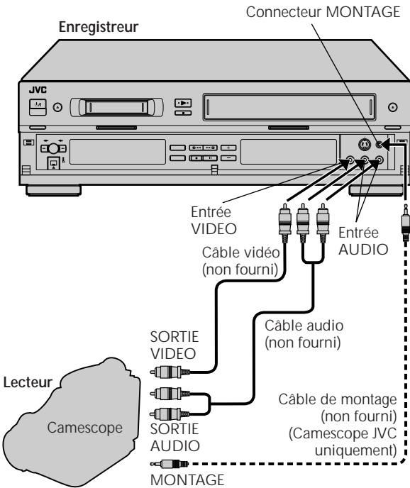
A Si le caméscope n'a pas de connecteur de sortie S-VIDEO ...
