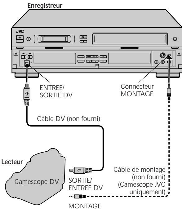
C Si le caméscope est muni d'un connecteur SORTIE/ENTREE DV ...
